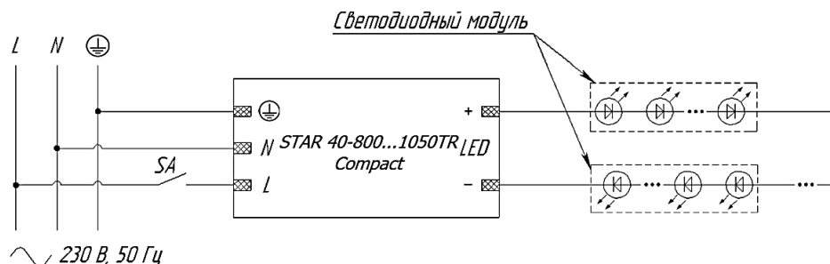
Рисунок 2 – Схема подключения источника
