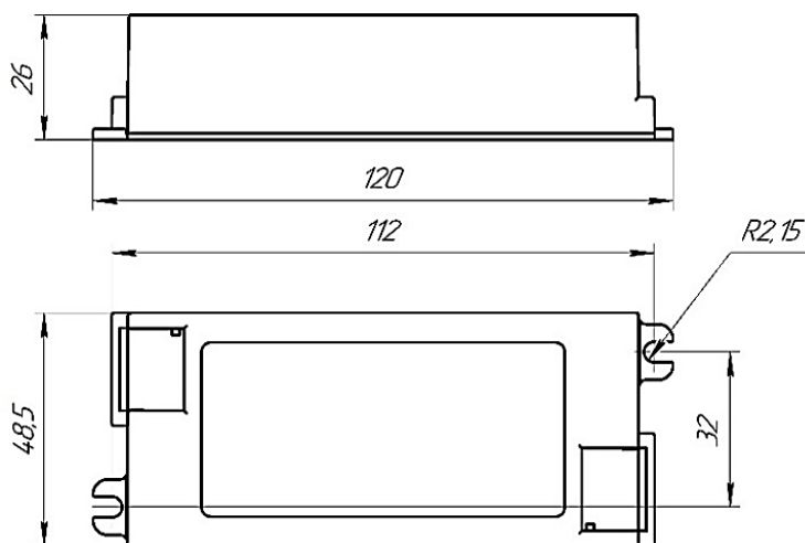
Рисунок 1 – Габаритные и установочные размеры
